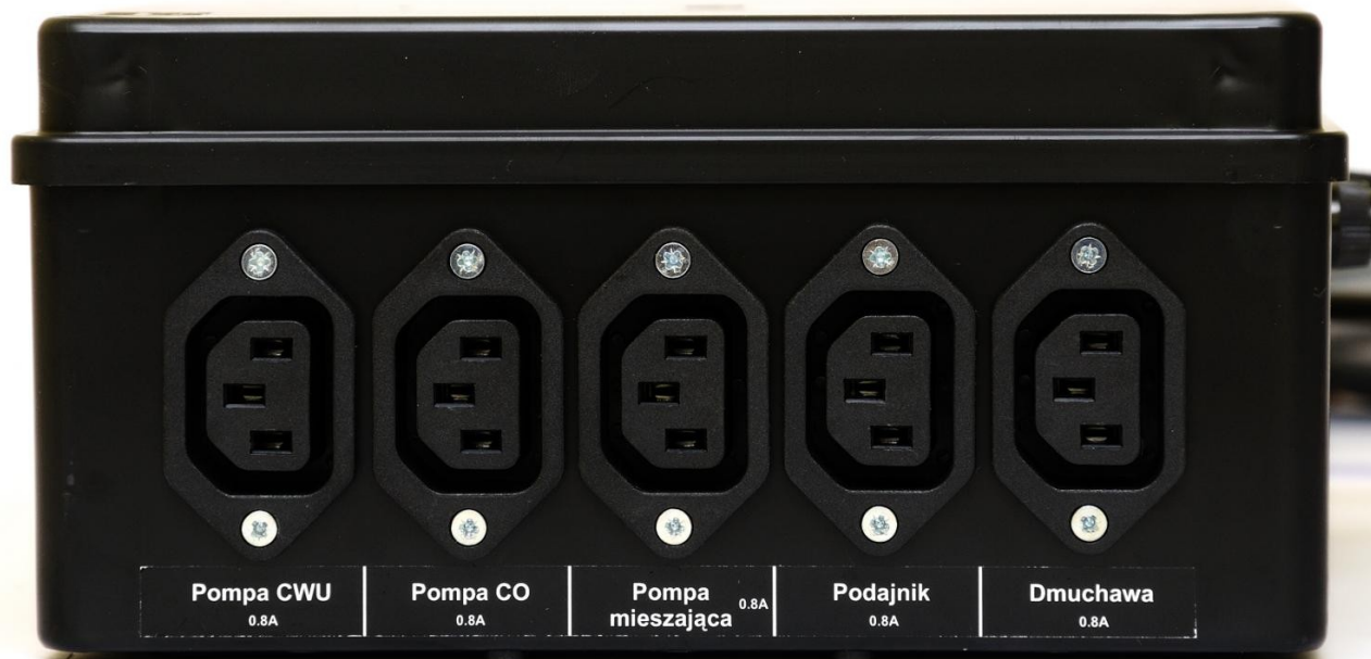
Иллюстрация 4: Стенка корпуса с выходами мощности
