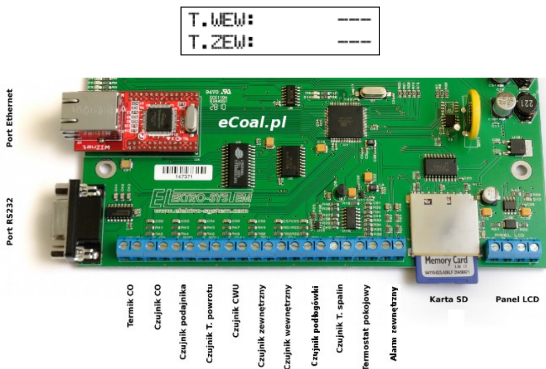
Иллюстрация 3: Зажимная планка для подключения датчиков
