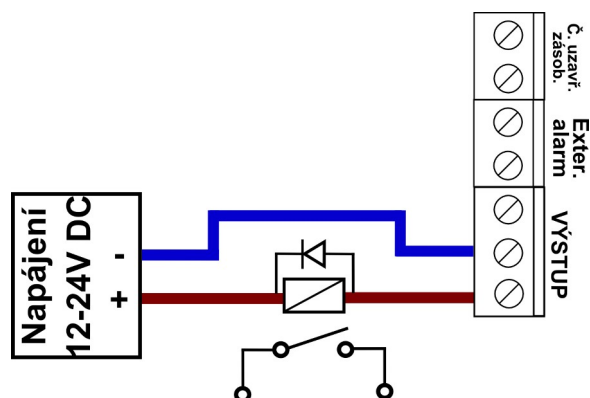
Obrázek 13: Připojení přídavného alarmu na výstup alarmu
