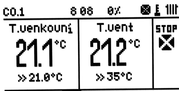
Obrázek 9: Obrazovka okruhu ÚT.1
