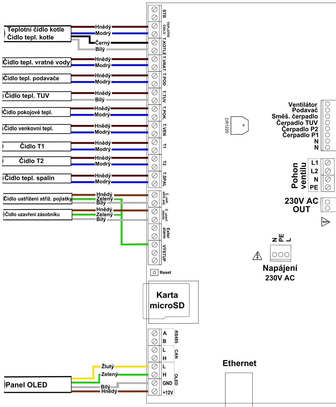
Obrázek 2: Svorkovnice pro zapojení čidel
