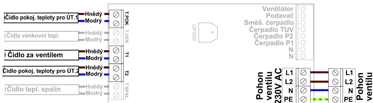
Obrázek 16: Zapojení pohonu ventilu a pokojových čidel pro okruh ÚT.1.
