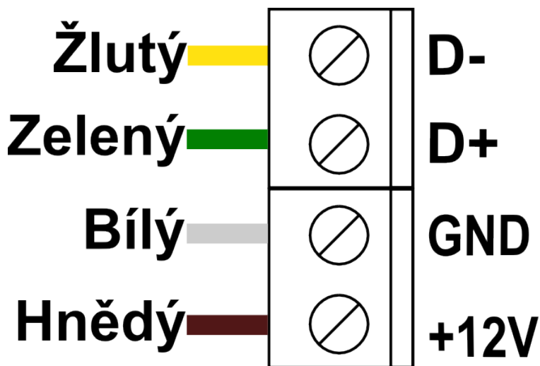
Obrázek 1: Zapojení panelu Standard
